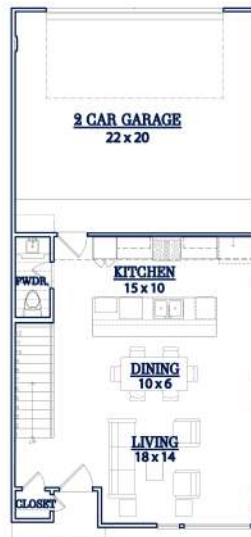
UNIT A5 - FIRST FLOOR SCALE: 1/4" = 1'-0"
